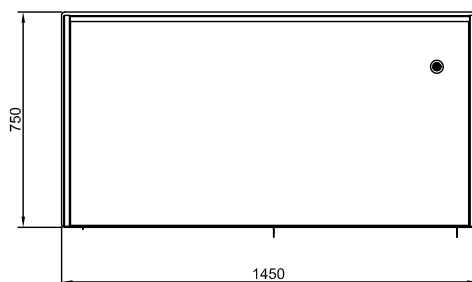
Boven aanzicht
